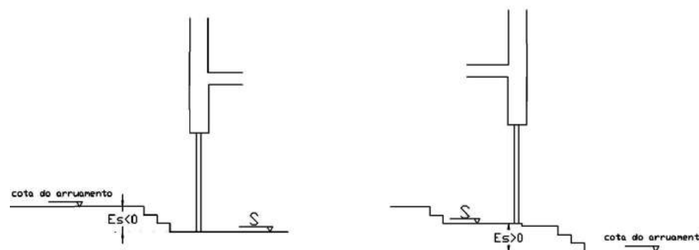
Figura 3 b - Cota de soleira; Elevação da soleira
